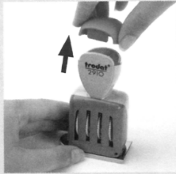
Einstellen des Datums auf der Höhe der Textplatte
